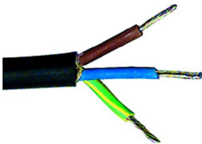
3x1,5mm 2
